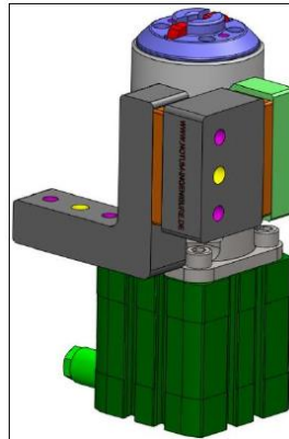
Prozesssichere Unterzugspanneinheiten
